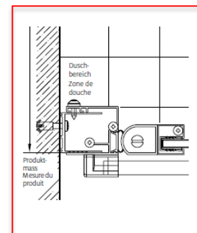
Montage bodeneben Montage à fleur de sol
